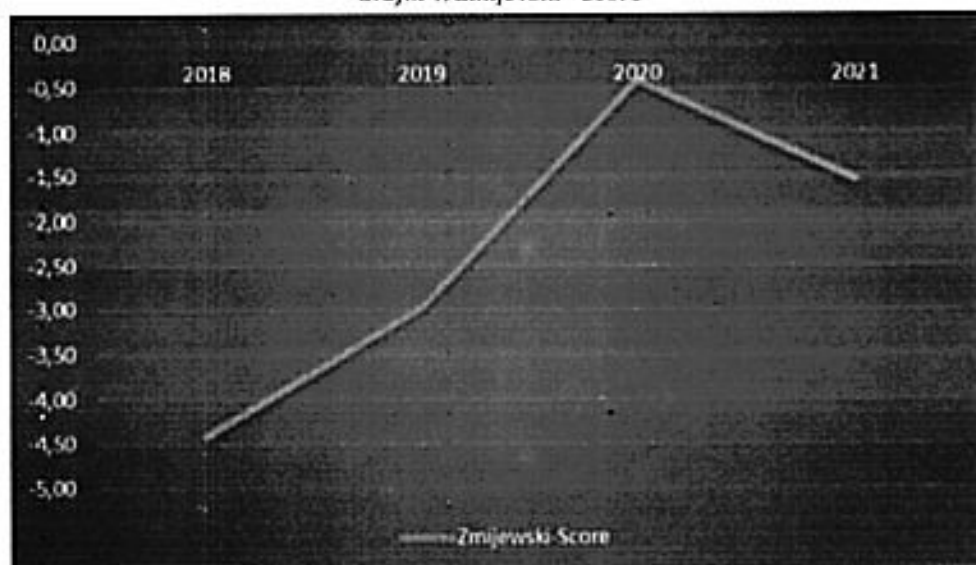
Grafik 4. Zmijevski - Score
